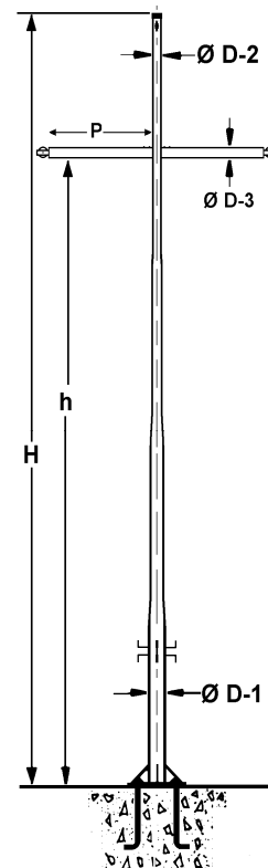
MB - 103 B
