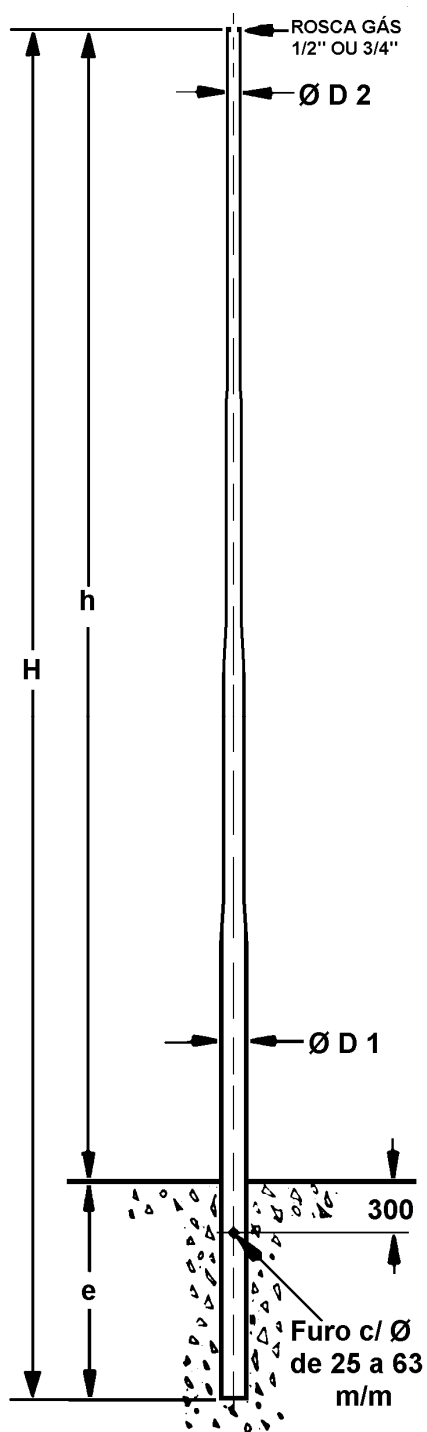
PR – 100 ENGASTADO
