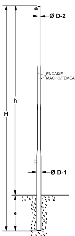
MB - 100
