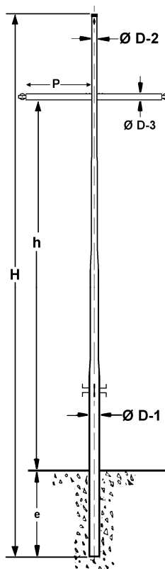
MB - 103
